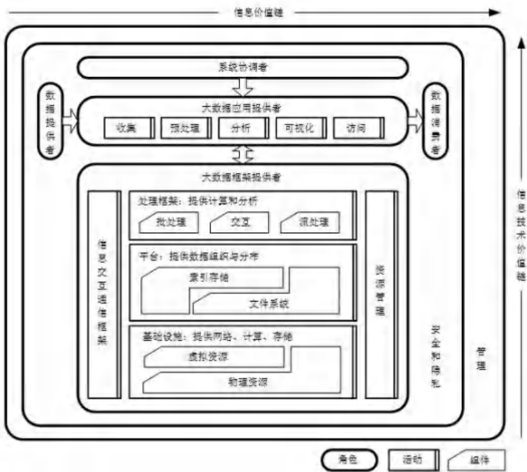
图 3-1 大数据参考架构图
